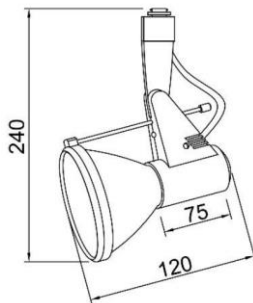
Dimensiones (mm)
